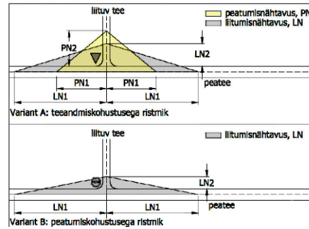
Joonis 1. Nähtavusala sametasandilisel ristmikul.
